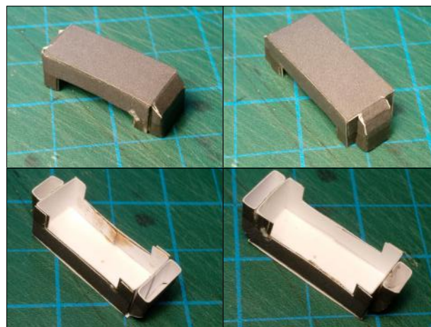
Τεμάχιο / Piece 3b συναρμολόγηση στο τεμάχιο 3a Βήμα 2. Κόλληση πλαινών assembling into piece 3a Step 2. Sides gluing
