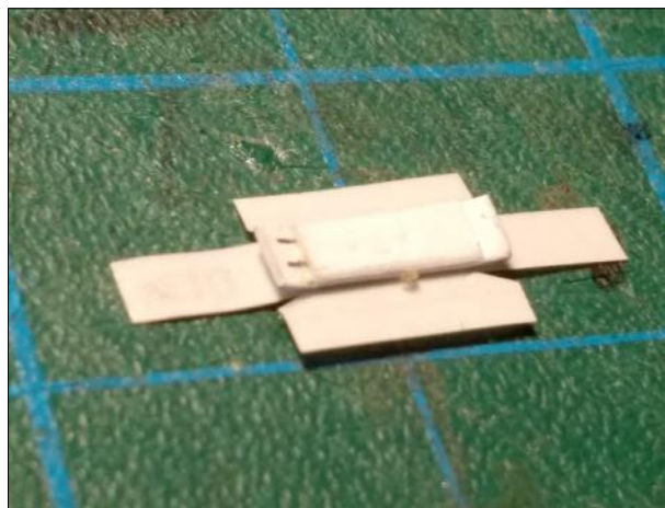
D13. Αεραγωγοί οροφής - Εναλλακτική Α' Τελική συναρμολόγηση - βημα 1 Κόλληση κομματιών D13a/b στο αυτοκόλλητο D13c D13. Roof air vents - Alternative A' Final assembly - step 1 Placing of pieces D13a/b into self-adhesive D13c
