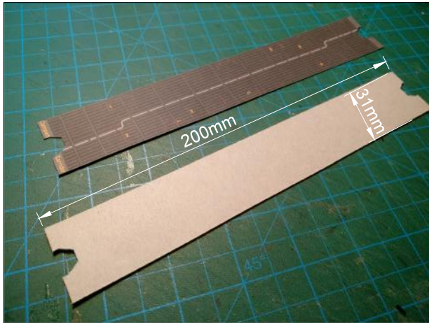
E1. Κομμάτι E1- κοπή Χρήση κομματιού E1 ως πατρόν και κοπή σε χαρτόνι πάχους 1mm E1. Piece E1 - cutting Use piece E1 as a template and cut into 1mm thick cardboard
