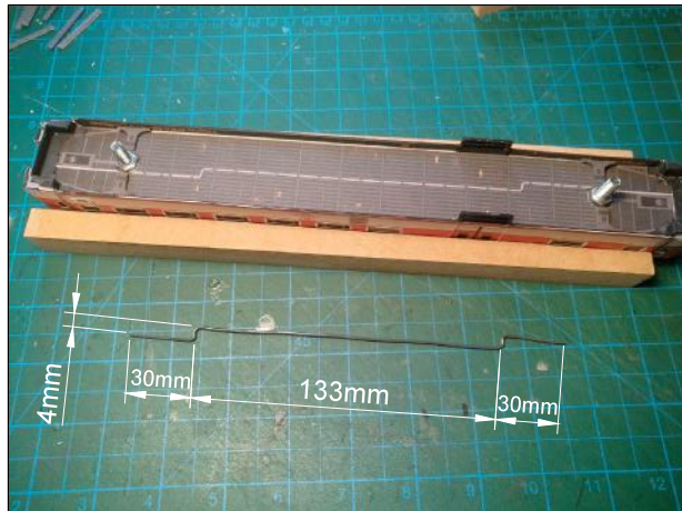
Ε3. Κατασκευή σωλήνας ατμού (προαιρετικό) Διαμόρφωση σωλήνας και βαφή. E3. Steam pipe construction (optional) Forming of the pipe and painting.
