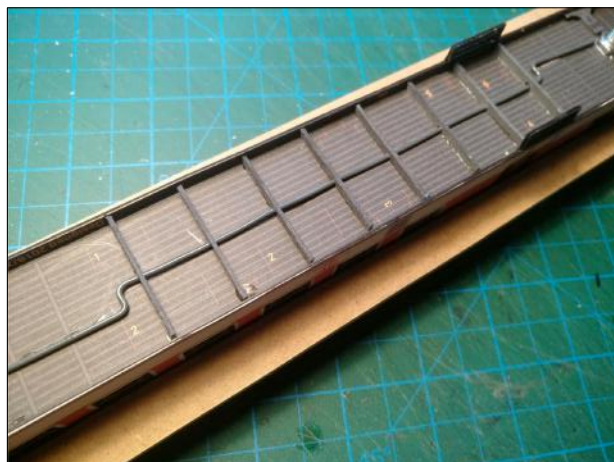
Ε4. Κατασκευή κάθετων δοκών πατώματος Κόλληση στο πάτωμα του βαγονιού E4. Floor vertical beams construction Gluing into wagon floor
