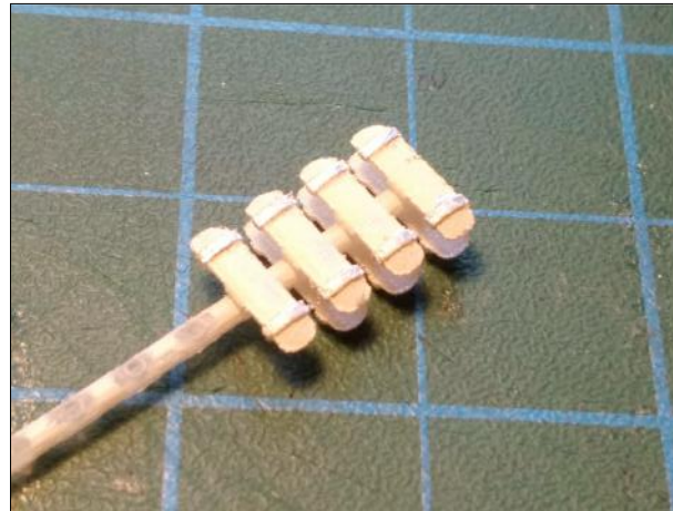
D13. Αεραγωγοί οροφής - Εναλλακτική Β' Αντικείμενο απο 3D εκτύπωση Προετοιμασία και βαφή D13. Roof air vents - Alternative B' 3d printed piece Preparation and painting
