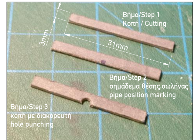
Ε4. Κατασκευή κάθετων δοκών πατώματος Κοπή 8 τεμαχίων 31x3mm από χαρτόνι 1mm. (Βήματα 2 και 3 μόνο αν κατασκευαστεί η σωλήνα ατμού). E4. Floor vertical beams construction Cut 8 pieces 31x3mm out of 1mm cardboard. (Steps 2 and 3 only with steam pipe construction)
