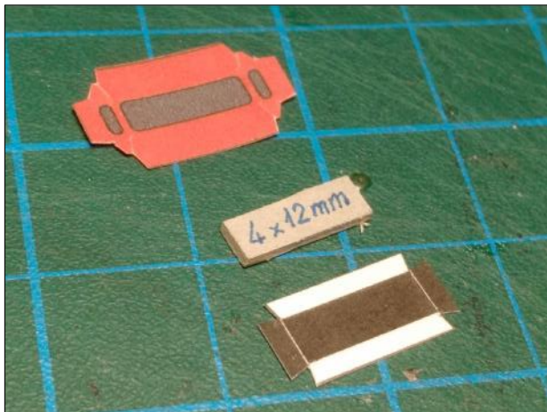
D12. ΜΟΝΟ ΓΙΑ ΟΧΗΜΑΤΑ ΣΚΕΥΟΦΟΡΟΥΣ - BDms παράθυρο προισταμένου - κοπή κομματιών D12a, D12b. Κοπή κομματιού διαστάσεων 4x12mm από χαρτόνι πάχους 1mm. D12. FOR BDms BAGGAGE VANS ONLY conductor's window - cutting of pieces D12a, D12b. From 1mm thick cardboard cut out a piece with dimensions 4x12mm
