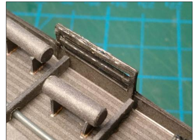
D17. ΜΟΝΟ ΓΙΑ ΟΧΗΜΑΤΑ ΣΚΕΥΟΦΟΡΟΥΣ - BDms κόλληση στο μοντέλο D17. FOR BDms BAGGAGE VANS ONLY gluing into model
