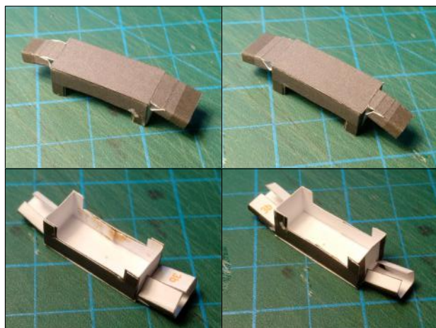
Τεμάχιο / Piece 3b συναρμολόγηση στο τεμάχιο 3a Βήμα 1. Κόλληση κατω επιφανειας assembling into piece 3a Step 1. Gluing bottom surface
