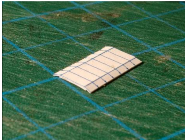
D13. Αεραγωγοί οροφής - Εναλλακτική Α' Κόλληση κομματιών D13a και D13b D13. Roof air vents - Alternative A' Gluing of pieces D13a and D13b
