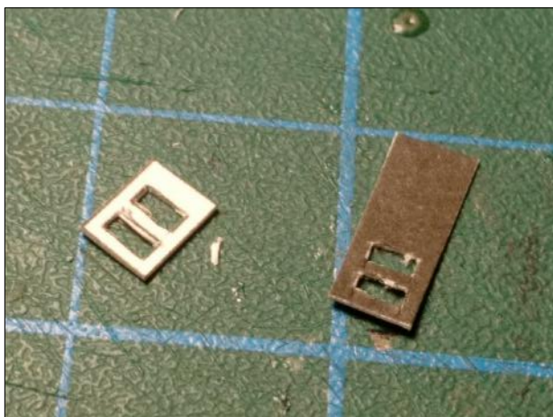
D17. ΜΟΝΟ ΓΙΑ ΟΧΗΜΑΤΑ ΤΑΧΥΔΡΟΜΕΙΑ - Post-m ενισχυτικά σκαλοπατιών - κοπή D17. FOR Post-m MAIL VANS ONLY steps reinforcing pieces - cutting
