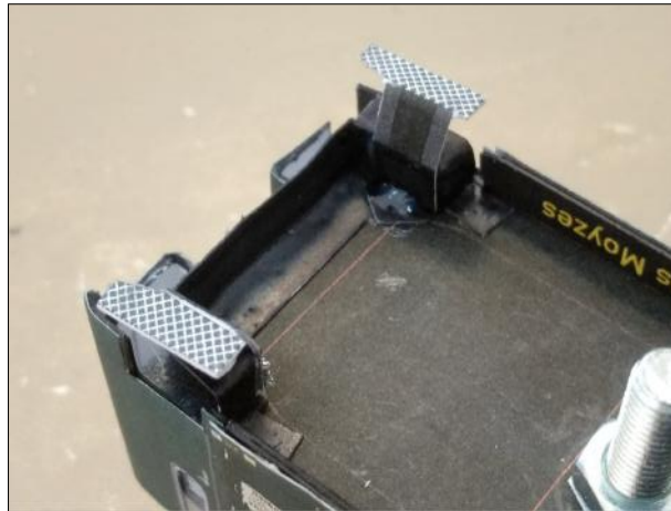
τελική συναρμολόγηση (οψη 2) final assembly (view 2)
