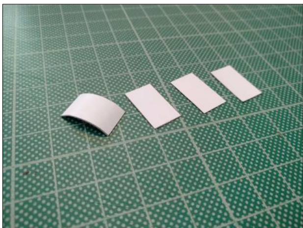
D12. Καλύμματα οροφής - κοπή και καμπύλωση D12. Roof covers - cutting and bending
