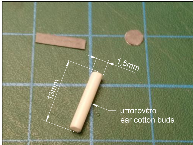
D14B. Αεραγωγός οροφής - MONO TAXYΔΡΟΜΕΙΑ Κοπή χάρτινων τεμαχίων Κοπή τεμαχίου μήκους 13mm από μπατονέτες D14B. Roof air vent - ONLY POST VANS Cut paper pieces Cut a piece from ear cotton buds with length 13mm
